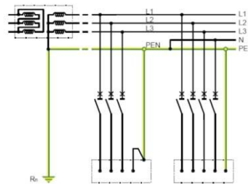
TN-C-S sistem
